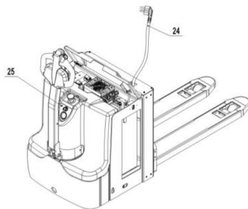
Рис.19: Зарядка аккумулятора встроенным зарядным
