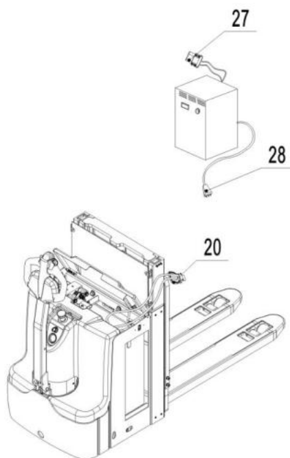
Рис.17: Зарядка аккумулятора
