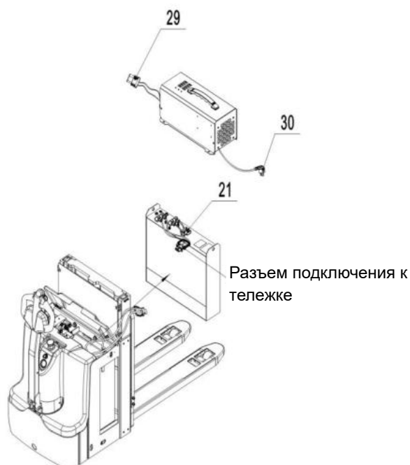
Рис.18: Зарядка литий-ионного аккумулятора
