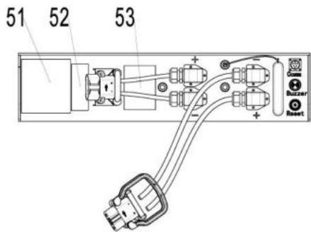
Рис. 11: Таблички аккумулятора
